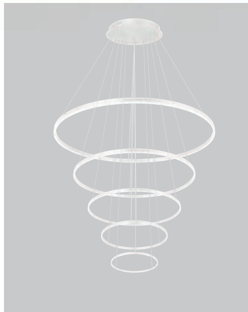
LU-MO-QUEEN-RC-B Blanco 110-220V 180 Watts D 100 + 800 + 600 + 400 + 200 mm 3 m de cable Aluminio Cálida/Natural/Frío
